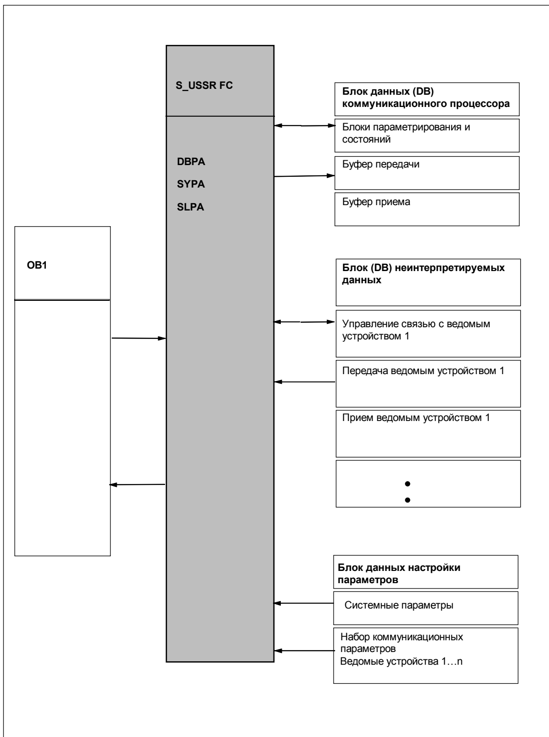
Рисунок 3–13 Структура программы
